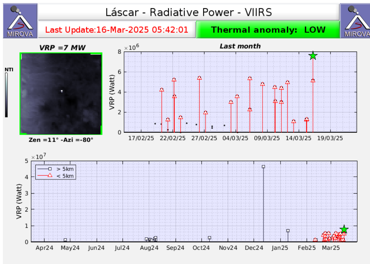
Figura 1. Reporte de la plataforma MIROVA que indica la anomalía térmica citada en este reporte. Se muestran los gráficos del Poder Radiativo según sensor VIIRS para el último mes (arriba) y el último año (abajo) ( https://www.mirovaweb.it/ ).
